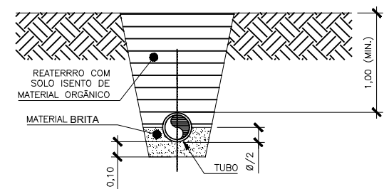
DETALHE TÍPICO DE ASSENTAMENTO DE TUBOS ESC.1:20
