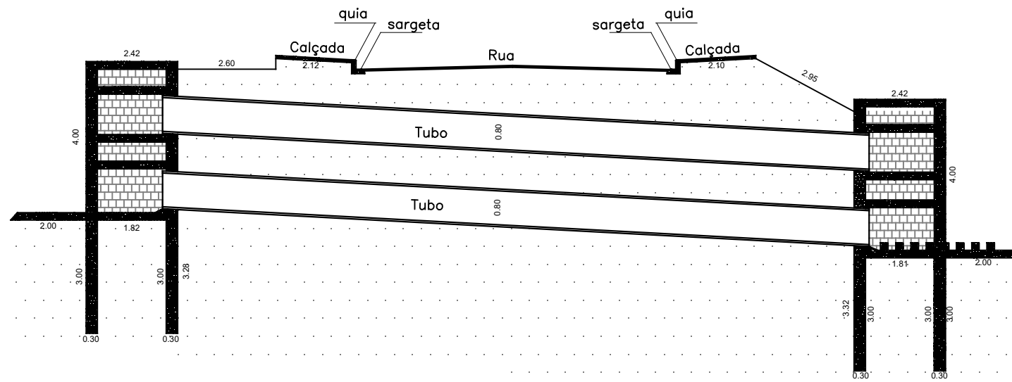
Corte Longitudinal -AA
