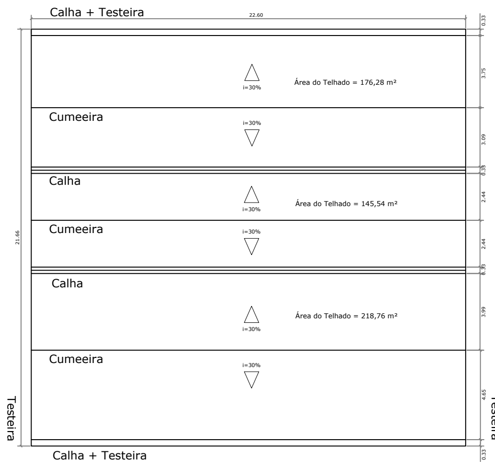
Planta do Telhado Esc.: 1/200
