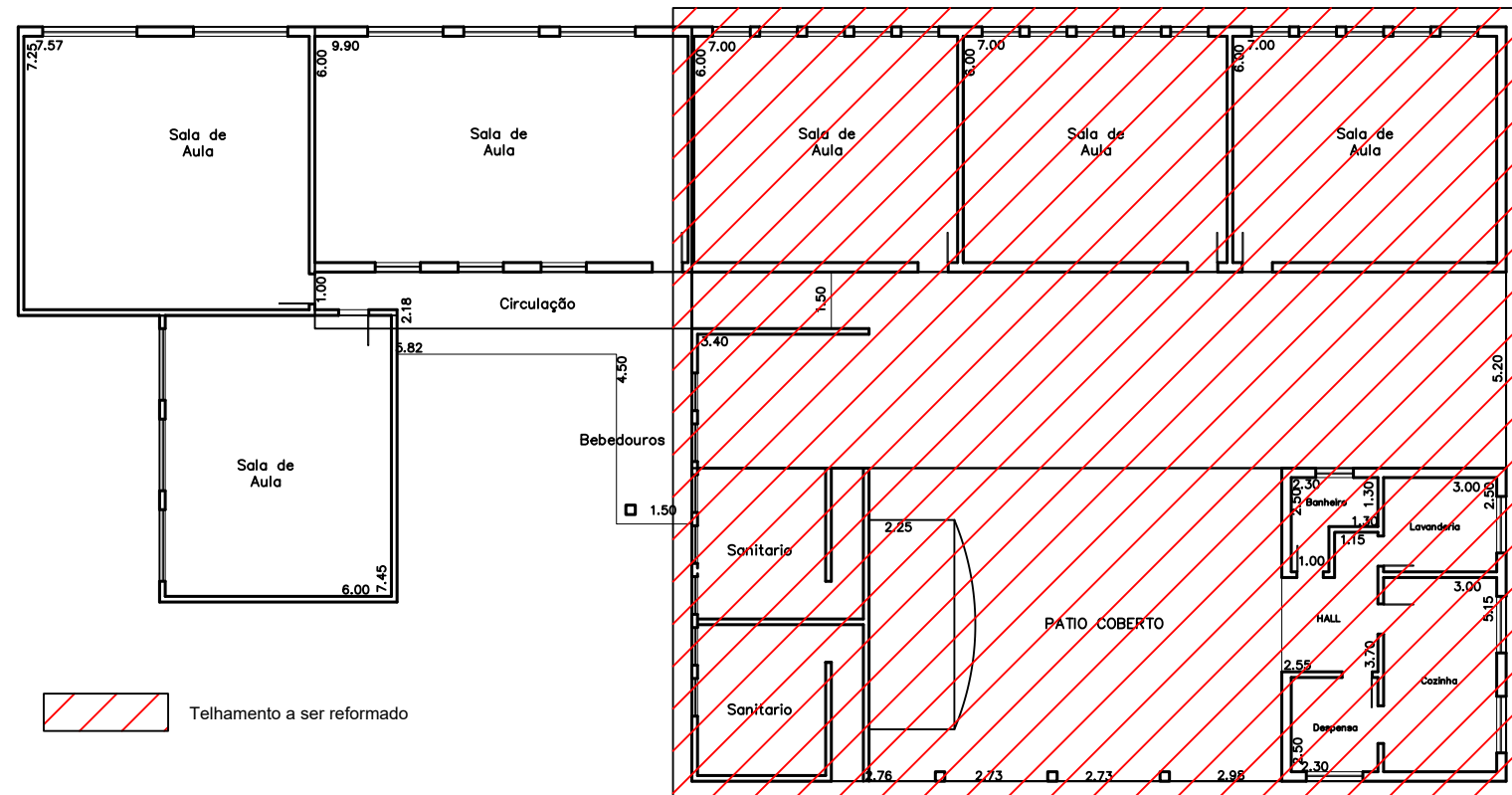
Planta da Escola Esc.: 1/200
